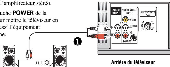
Amplificateur stéréo
